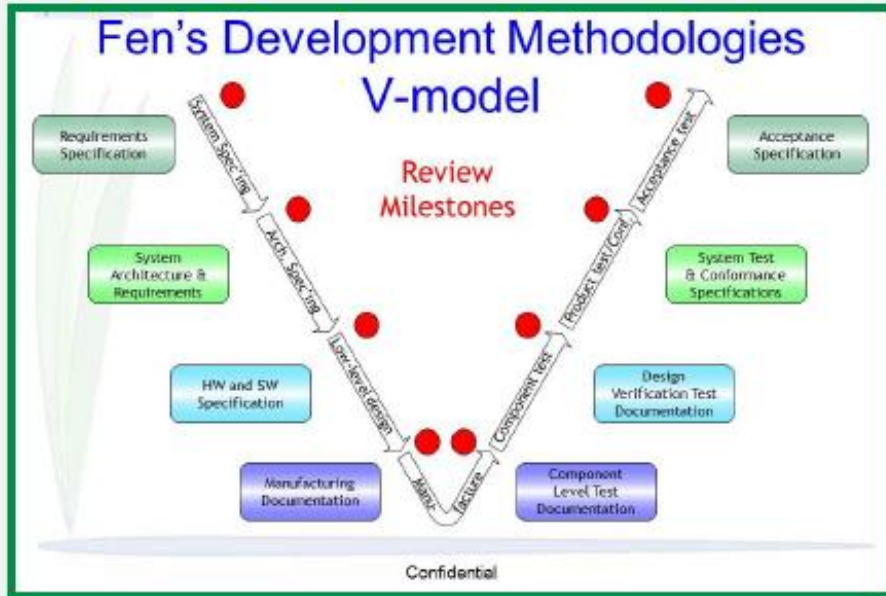
V-Model
